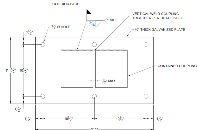
2 BASE PLATE - BP2 SCALE: 3" = 1'-0"
