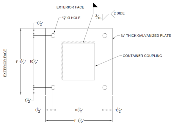
1 BASE PLATE - BP1 SCALE: 3" = 1'-0"
